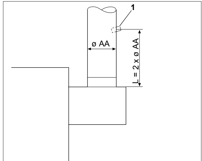
Рис. 31 Проведение замеров
