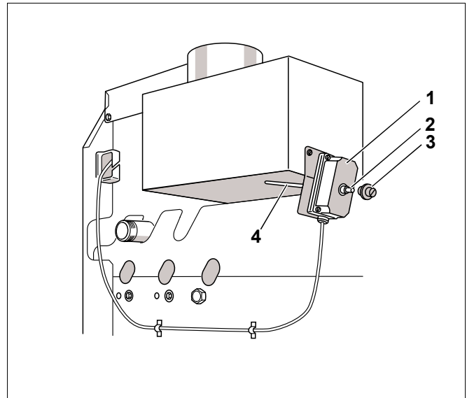
Рис. 35 Проверка системы контроля дымовых газов AW 10
