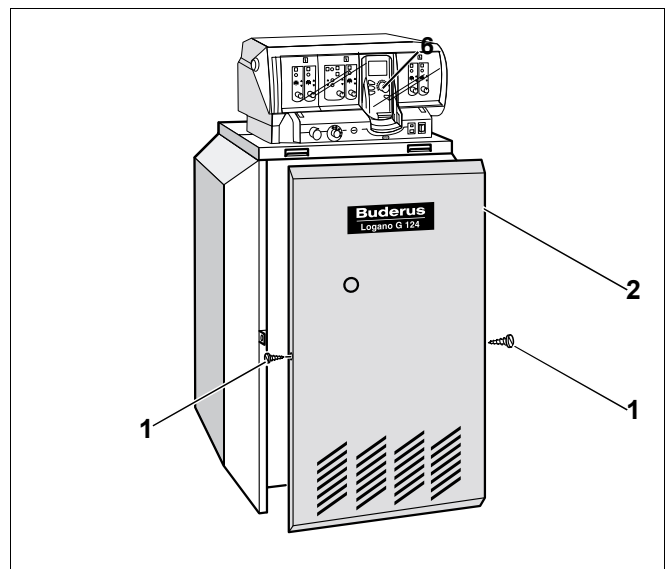
Рис. 36 Установка передней стенки котла
