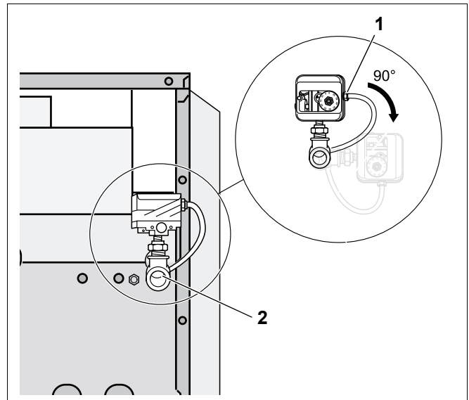
Рис. 23 Подключение газа
