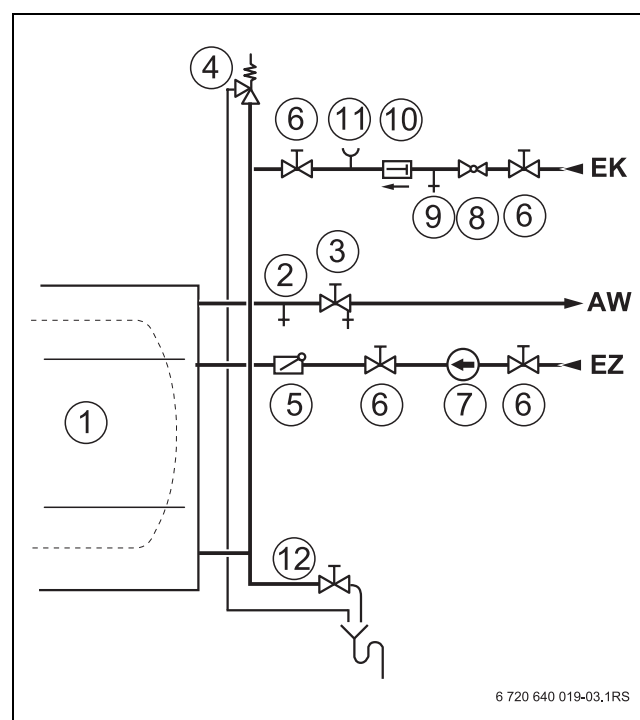
Рис. 6 Гидравлическая схема подключения бака
