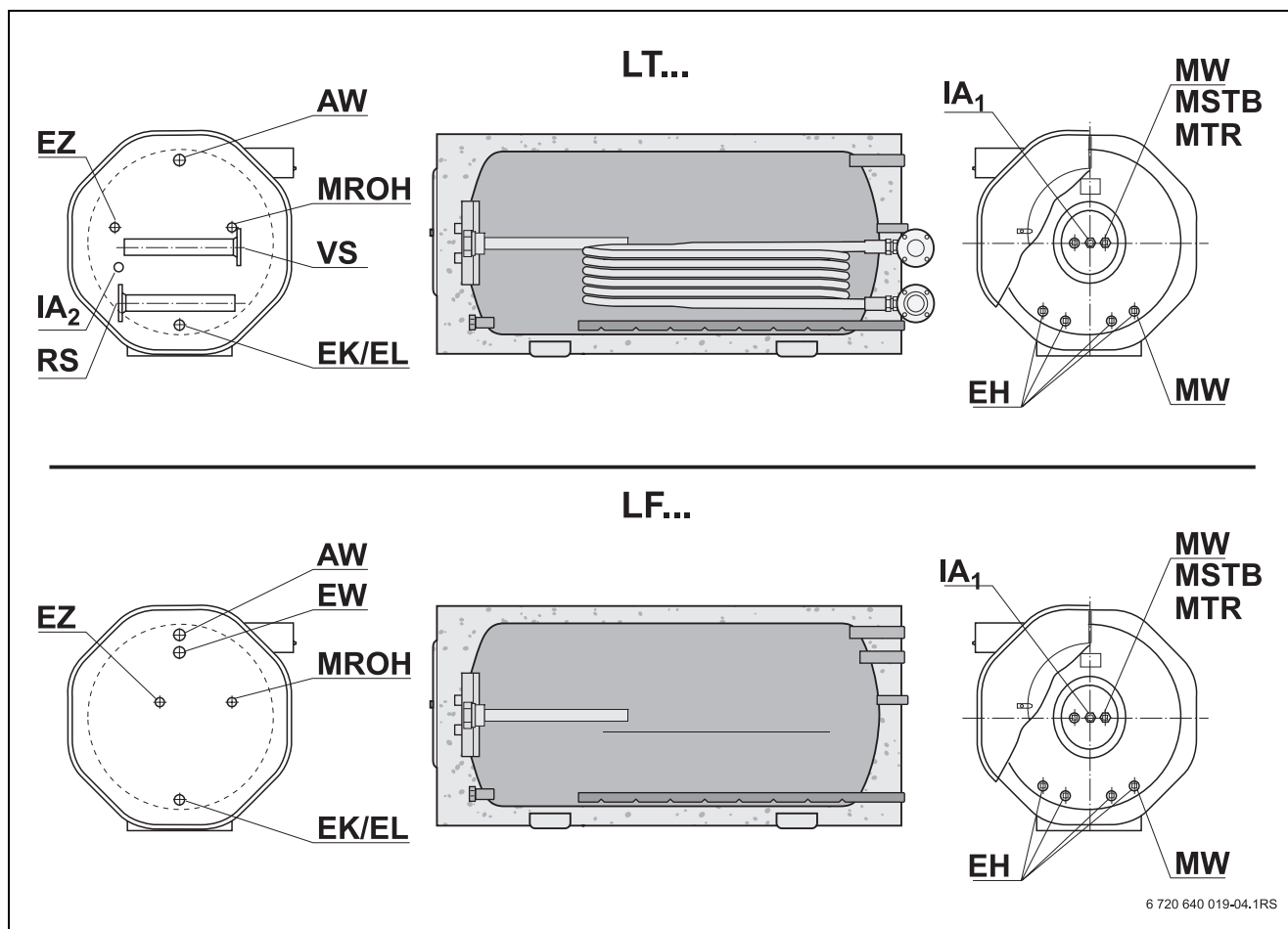
Рис. 1 Подключения LT/LF
