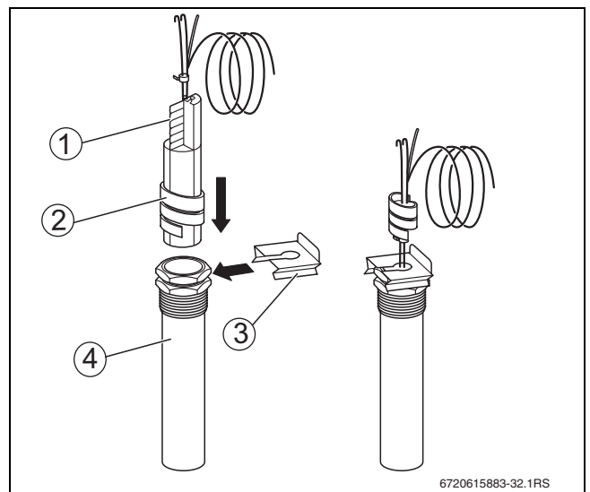
Рис. 19 Установка пластмассовой спирали в погружную гильзу
