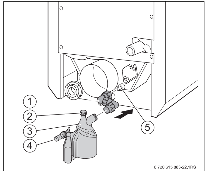
Рис. 27 Подключение линии отвода конденсата
