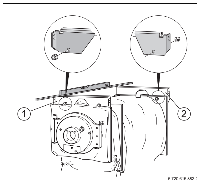
Рис. 7 Установка передней и задней траверс
