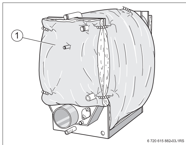
Рис. 6 Крепление теплоизоляции задней стенки
