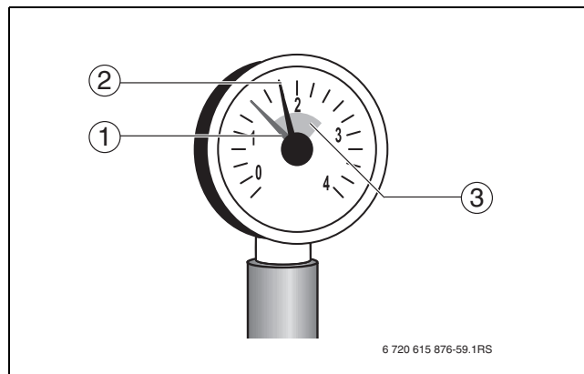
Рис. 34 Манометр для закрытых отопительных установок
