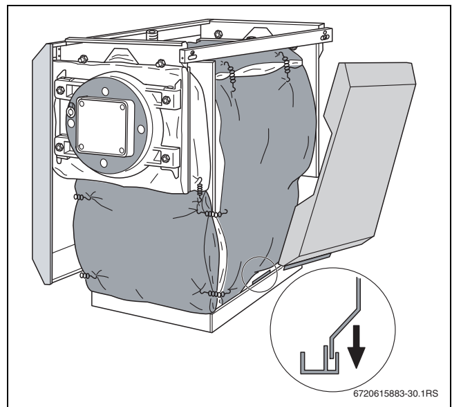
Рис. 12 Установка боковых стенок
