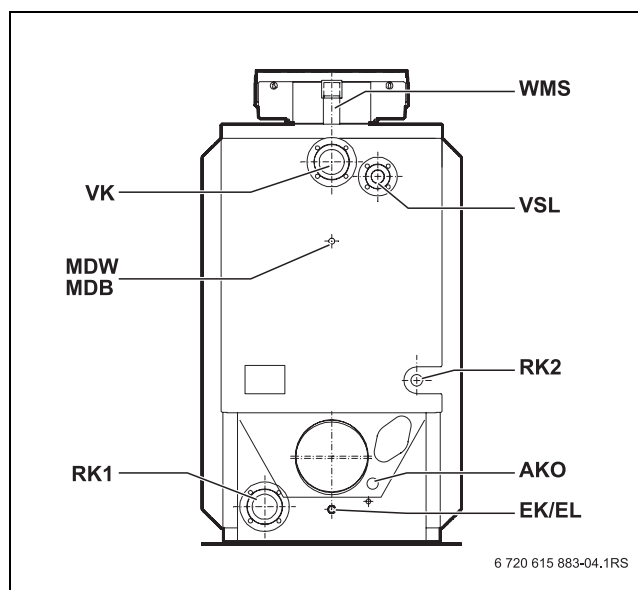
Рис. 5 Подключения на котле Logano plus SB615 Gas
