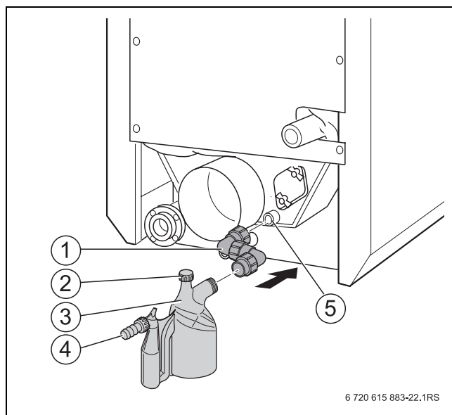
Рис. 27 Подключение линии отвода конденсата
