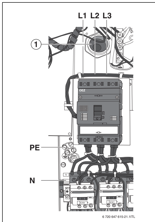
Рис. 8 Подключение сетевого провода 36—60 кВт (5-проводная сеть)
