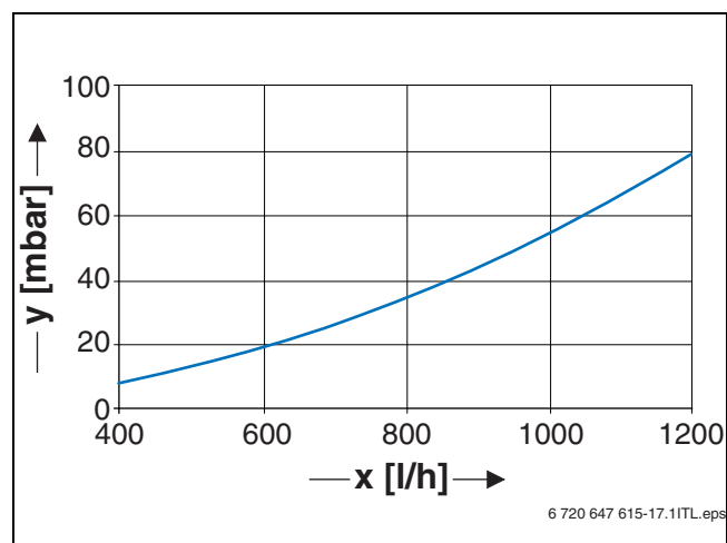
Рис. 42 Гидравлическое сопротивление Logamax E213 4 – 18
