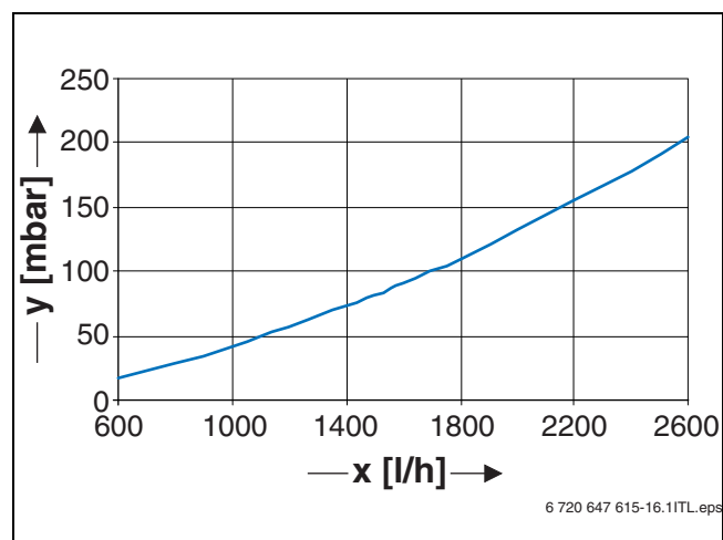
Рис. 41 Гидравлическое сопротивление Logamax E213 22 – 60
