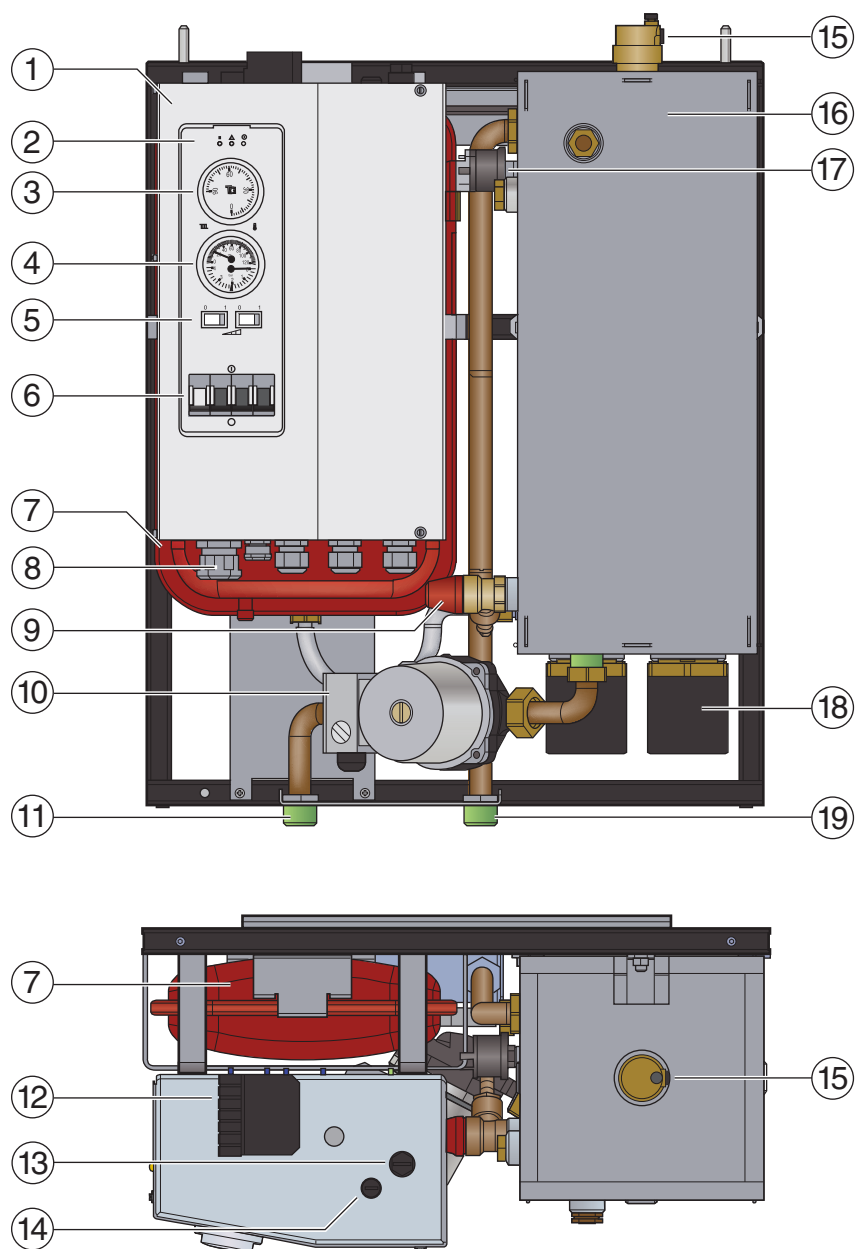
Рис. 1 Функциональные элементы котла
