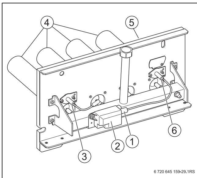
Сурет 53 Жанарғыны тазарту
