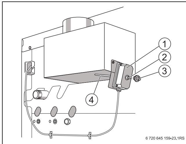
Сурет 41 AW 10 пайдаланылған газды бақылау жүйесін тексеру
