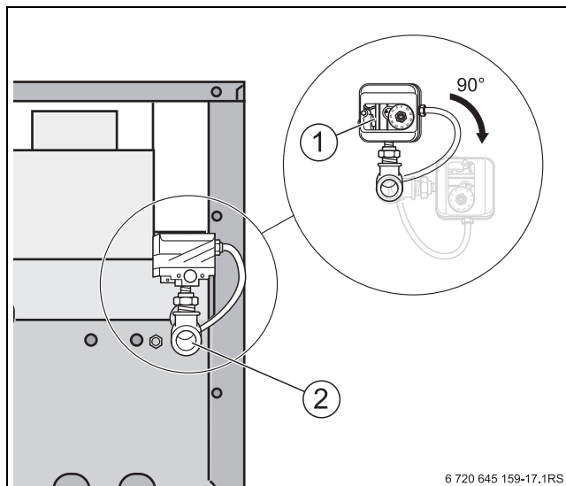
Сурет 10 Газды қосуды орындау
