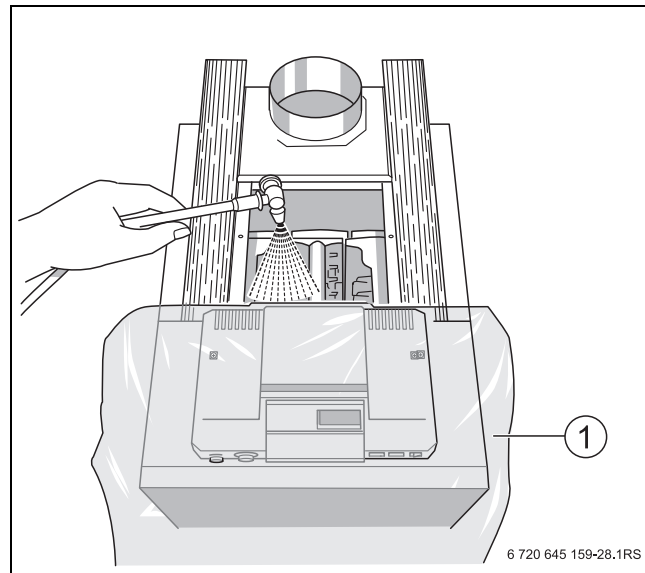
Сурет 52 Қазанды дымқыл шүберекпен тазарту
