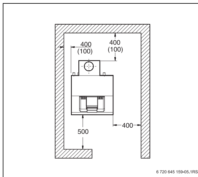
Сурет 7 Қабырғамен арадағы ұсынылатын қашықтық (өлшемдері мм-мен берілген, минималды қашықтар жақшаға алынған)
