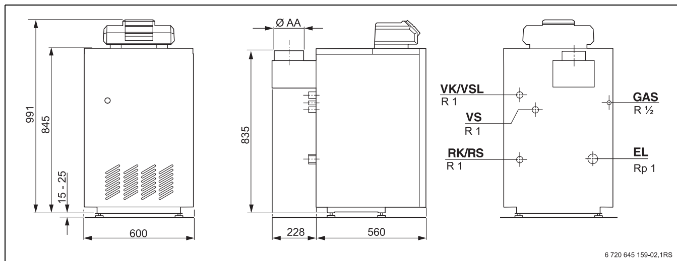
Сурет 3 Өлшемдері мен қосылымдары (өлшемдер миллиметрмен көрсетілген)
