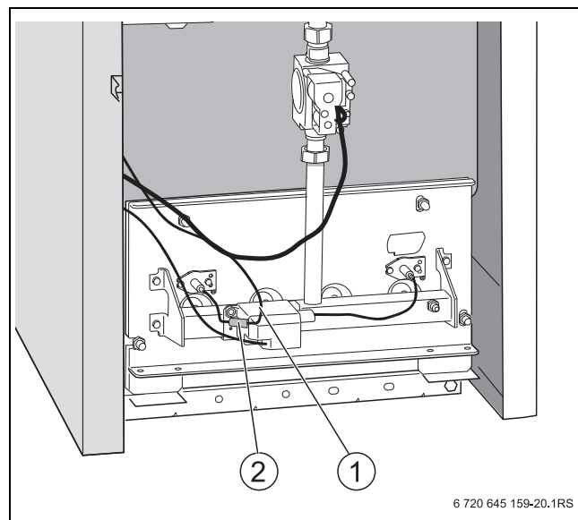
Сурет 38 Жанасу қорғанысын ажырату
