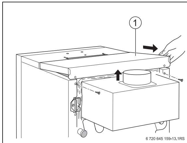
Сурет 16 Қазанның артқы қақпағын алу
