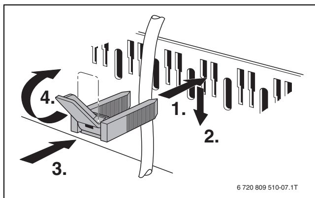
Сурет 23 Сымдарды кабель ұштықтарымен бекіту
