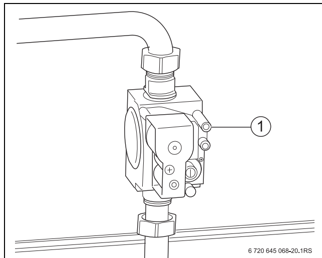
Сурет 31 Газ құбырын ауадан босату
