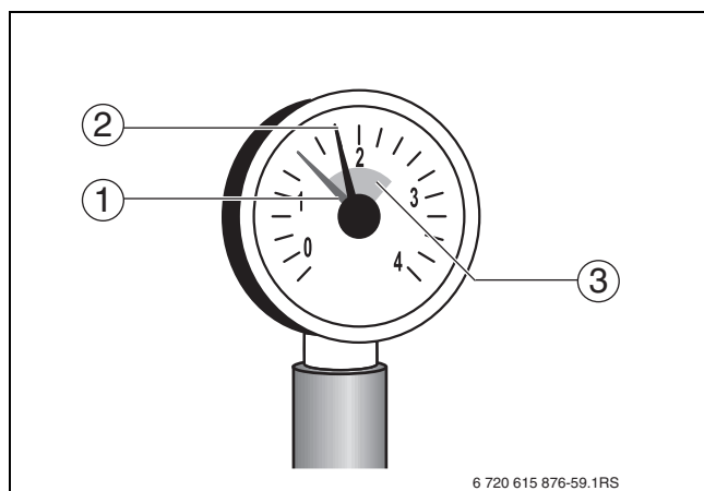
Сурет 14 Ажыратылған құрылғыларға арналған манометр
