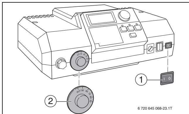
Сурет 33 Реттегіш құрылғыда жылыту қондырғысын қосыңыз (Logamatic 2000)
