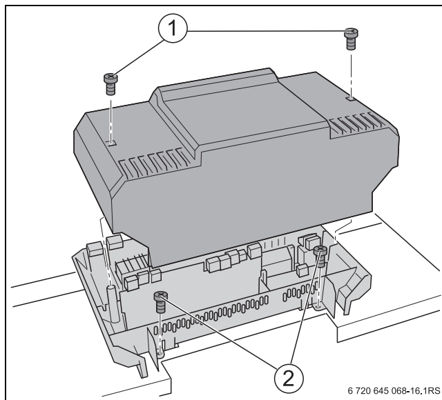
Сурет 18 Қабын алу
