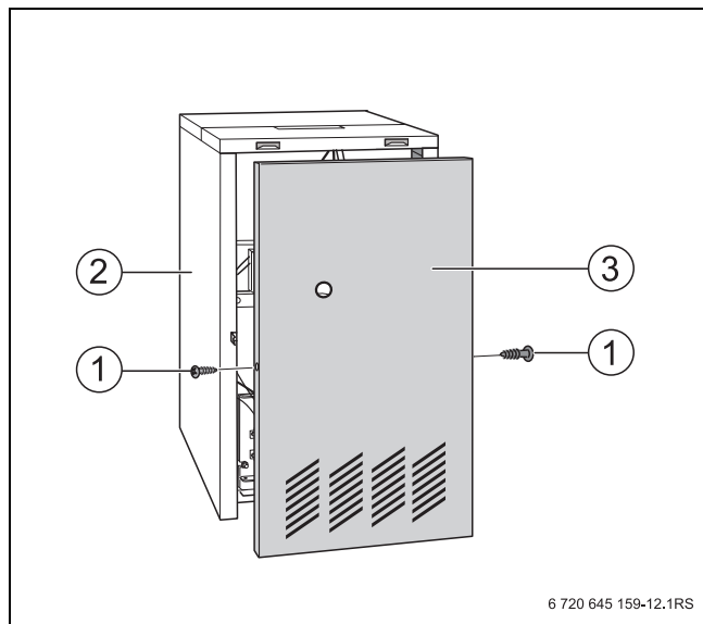
Сурет 15 Қазанның алдыңғы бөлігін ажырату
