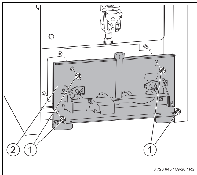
Сурет 50 Бекіту тетіктерін ажырату
