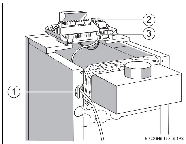
Сурет 22 Электр қосылымы желісін жалғау
