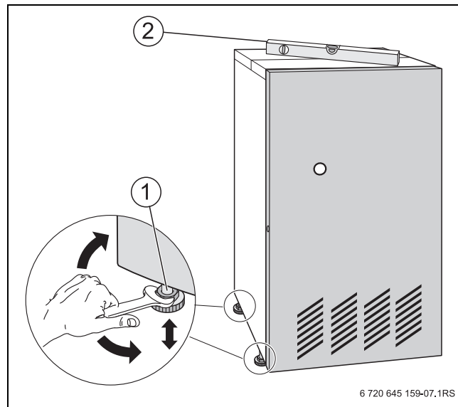
Сурет 9 Қазанды қою
