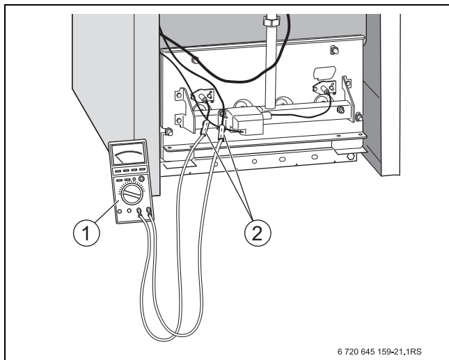
Сурет 39 Иондану ағынын өлшеу
