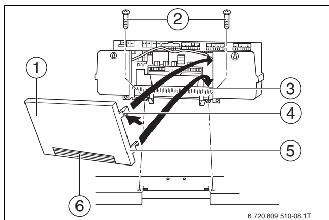
Сурет 25 Logamatic 4000 берік бұрап бекіту
