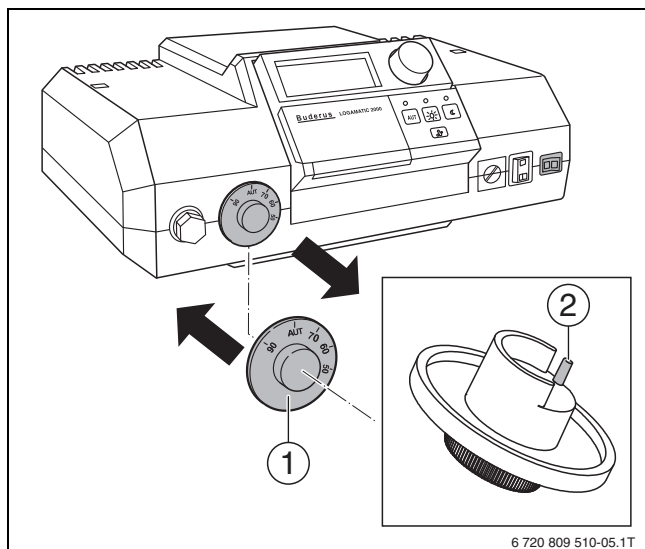
Сурет 26 Қазандағы температураны реттегішті тетікке алмастыру
