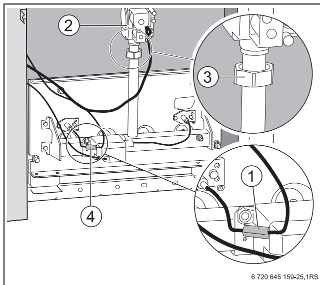
Сурет 49 Жанарғыны ажырату
