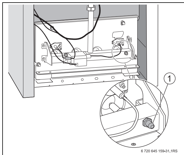
Сурет 48 Форсункалар қысымын өлшеу
