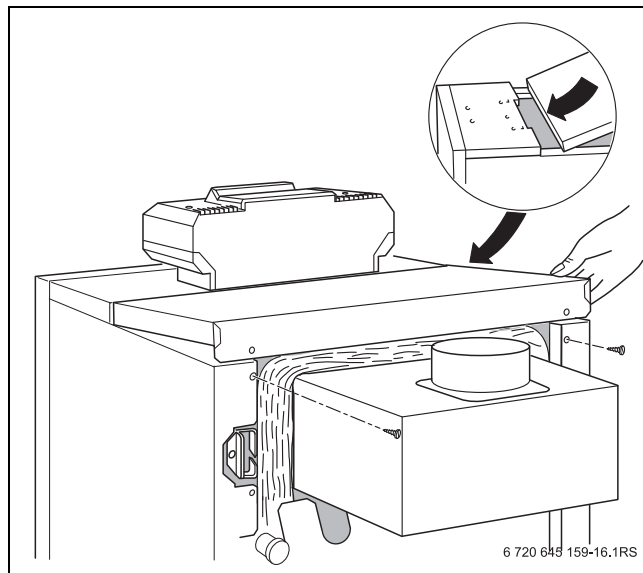
Сурет 28 Қазанның артқы қақпағын орнату
