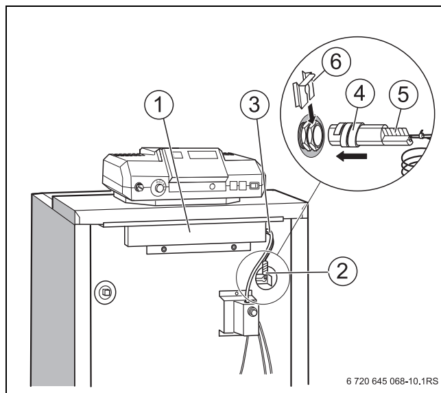
Сурет 21 Температура сезінгіш бумасын орнату
