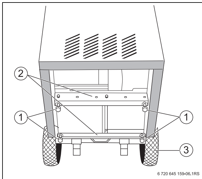
Сурет 8 Реттелетін аяқтарын тасымалдау көлігімен қою
