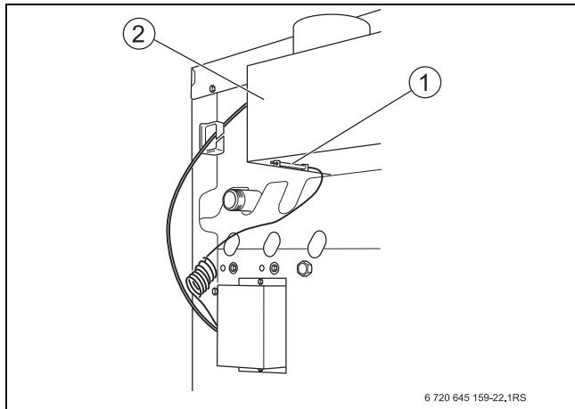
Сурет 40 AW 50 пайдаланылған газды бақылау жүйесін тексеру
