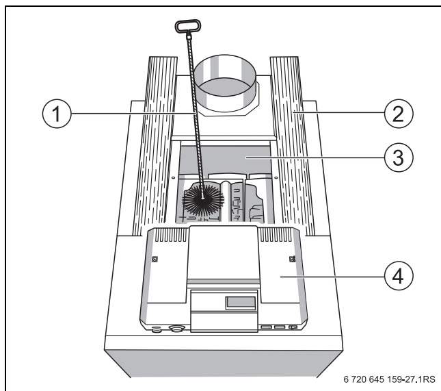
Сурет 51 Газ жеткізу жолдарын тазарту
