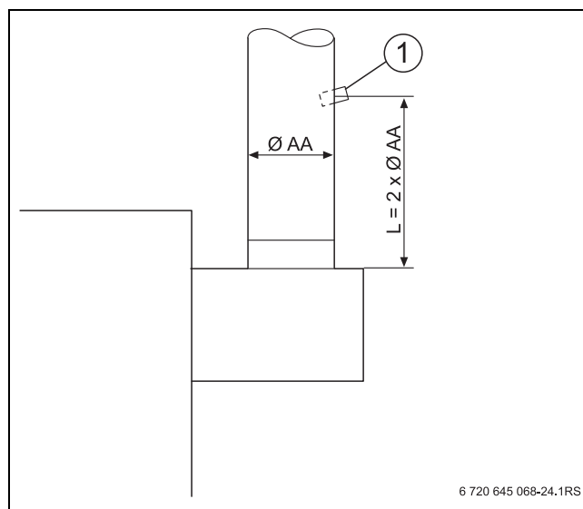
Сурет 37 Газ құбырындағы өлшеу орны
