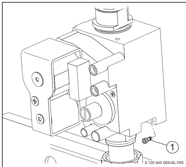
Сурет 57 Сұйықтық адаптерін орнату/шығару
