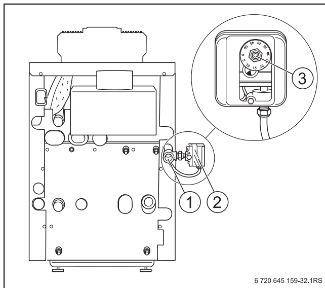
Сурет 55 Газ қысымын бақылау құралын орнату
