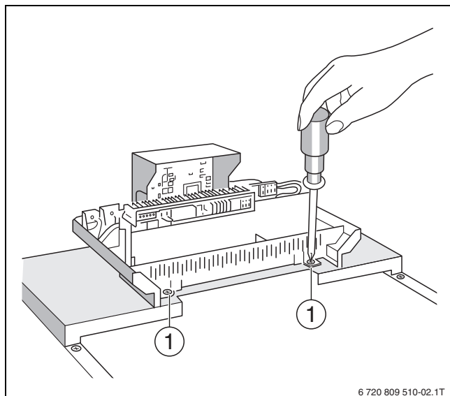
Сурет 20 Реттегіш құрылғына бұрап бекіту
