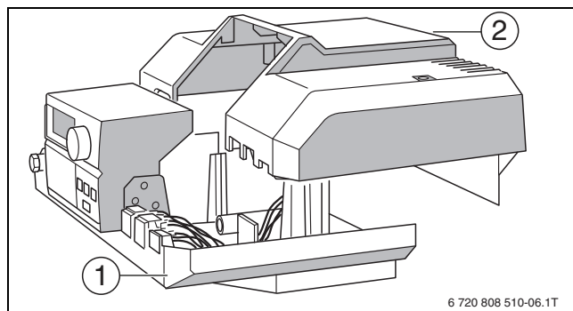
Сурет 27 Қысқыш қабын кигізу
