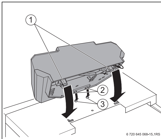
Сурет 17 Реттегіш құрылғыны орнату
