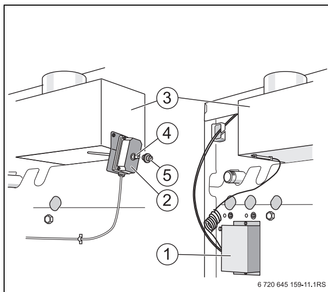
Сурет 13 Пайдаланылған газды бақылау жүйелері
