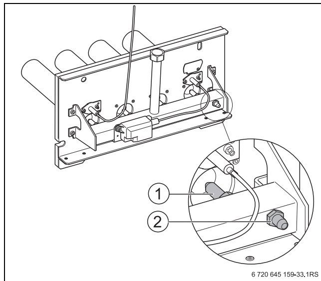
Сурет 58 Негізгі газ форсункаларын алмастыру
