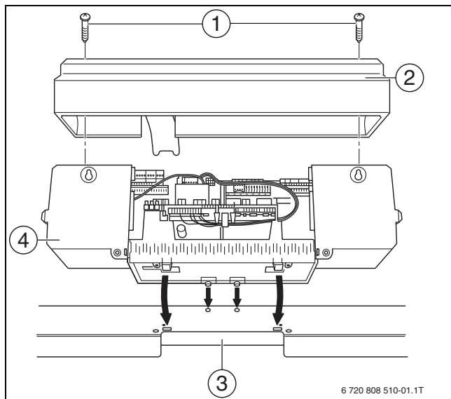
Сурет 19 Реттегіш құрылғыны ашу және кигізу
