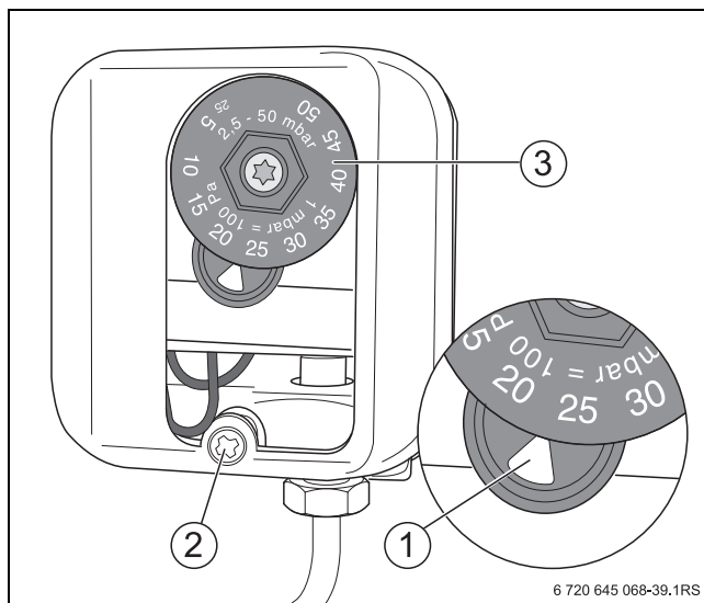
Сурет 56 Газ қысымын бақылау құралы
