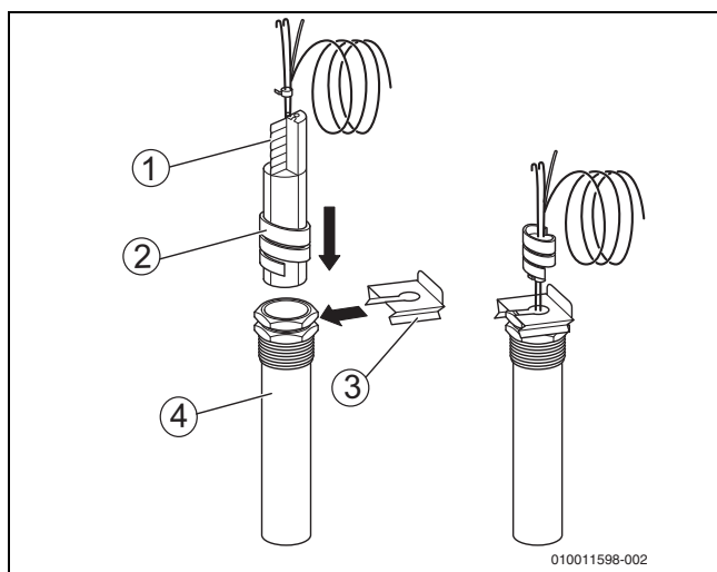
Рис. 7 Установка пластмассовой спирали в погружную гильзу@@
