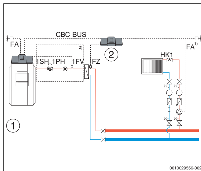
Рис. 35 Вариант 3: система управления низшего уровня без функции предварительного смешивания, с компенсацией потери тепла по датчику FZ, ограничением нагрузки и режимом нагрева при потерях тепла
