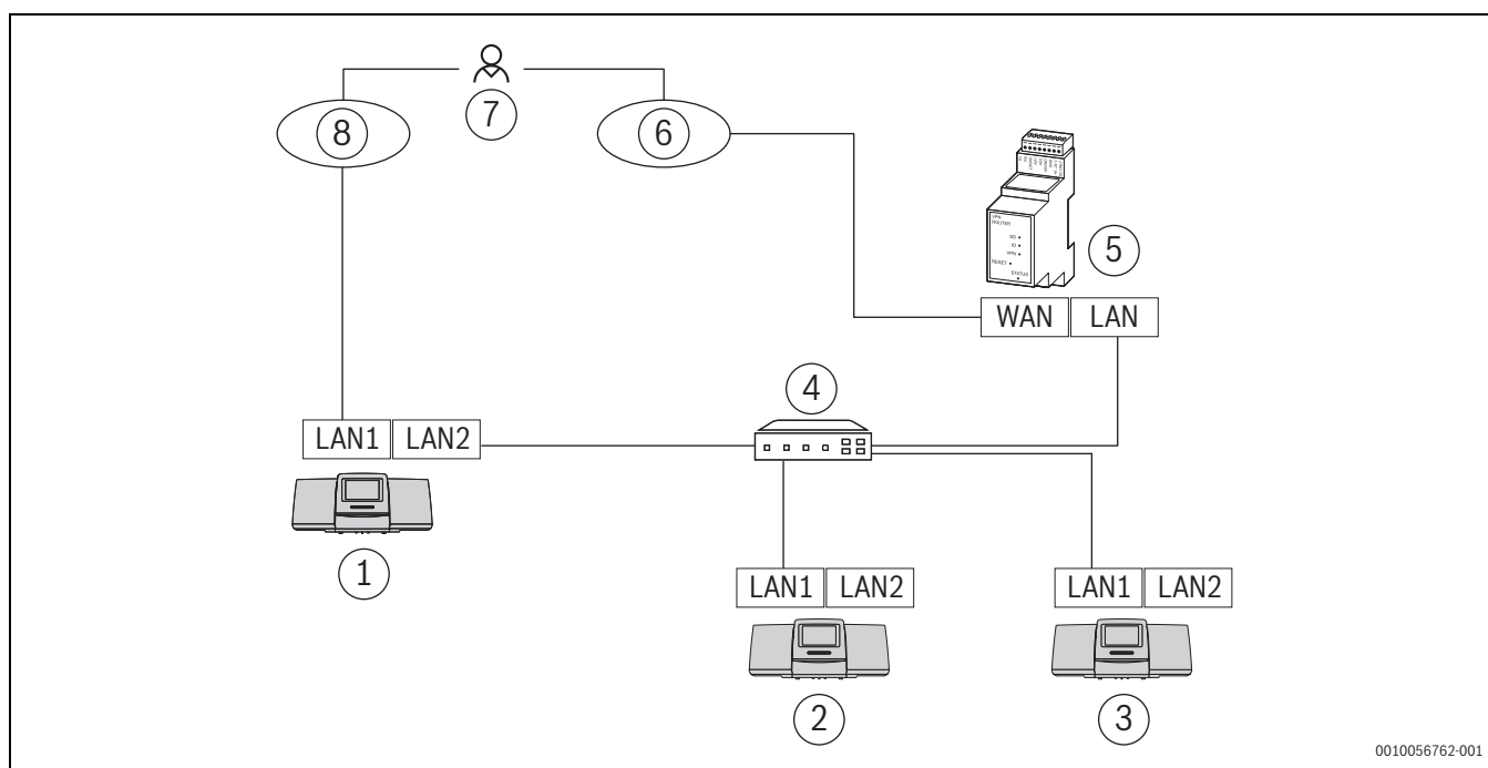
Рис. 47 Пример соединения нескольких систем управления с удаленным доступом и системы управления зданием
