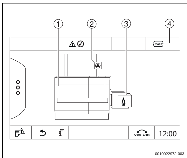
Рис. 58 Функциональные испытания Горелка
