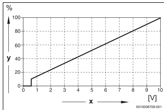
Рис. 29 Вход 0 ... 10 В Мощность
