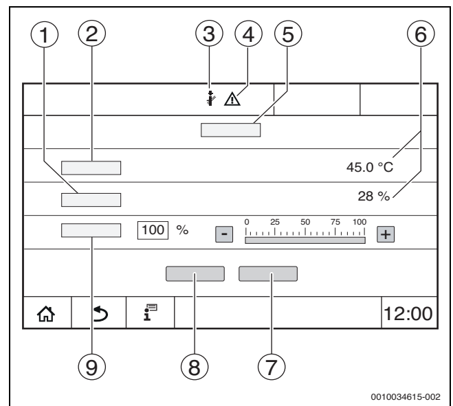
Рис. 21 Индикация Тест дымовых газов > настройки котла
