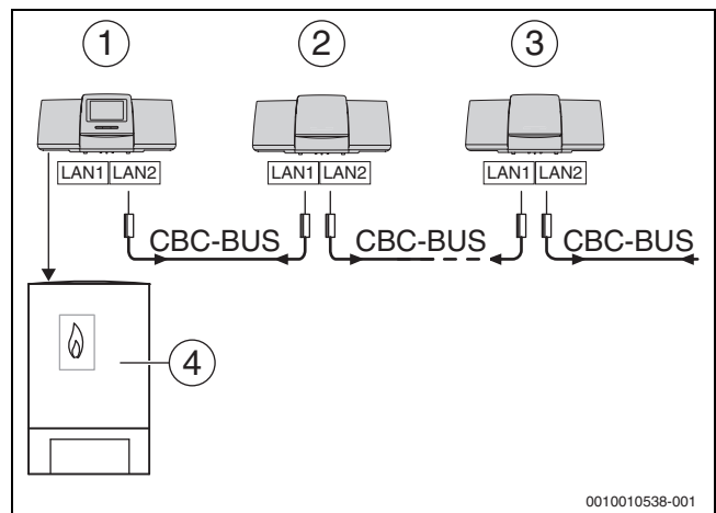
Рис. 46 Пример соединения нескольких систем управления
