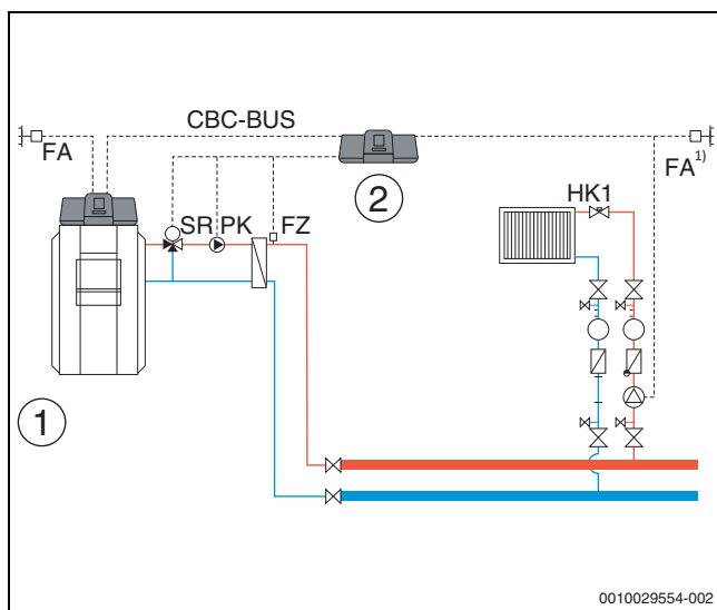
Рис. 33 Вариант 1: система управления низшего уровня с функцией предварительного смешивания, компенсацией потери тепла по датчику FZ и ограничением нагрузки
