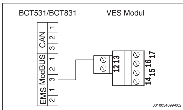
Рис. 37 Подключение системы управления к Модуль VES
