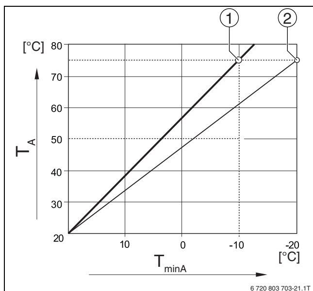
Рис. 27 Настройка отопительной кривой: угол наклона определяется расчётной температурой и минимальной наружной температурой
