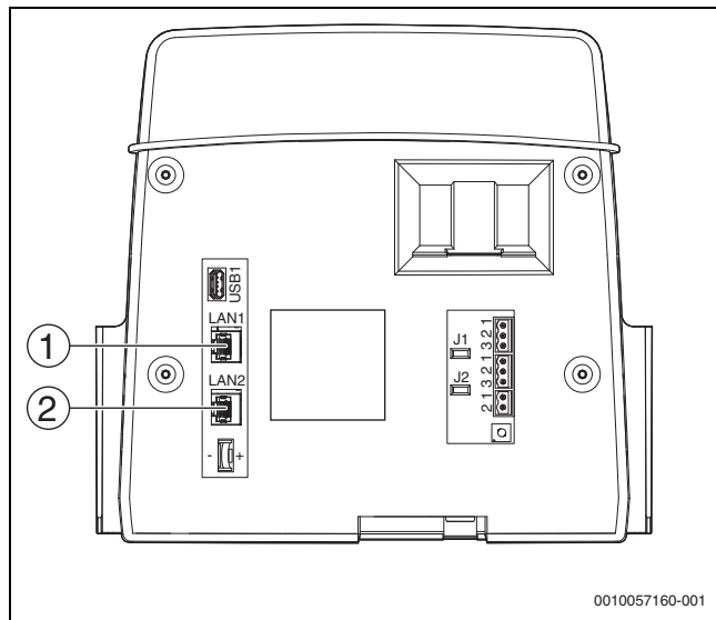
Рис. 45 Подключение для LAN1 и LAN2
