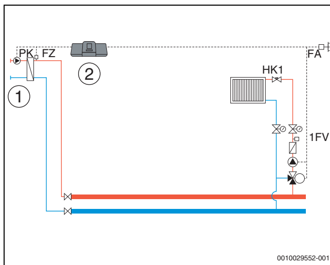
Рис. 31 Вариант 2: сторонний источник тепла без питающего насоса, ограничения нагрузки и компенсации потери тепла посредством FZ
