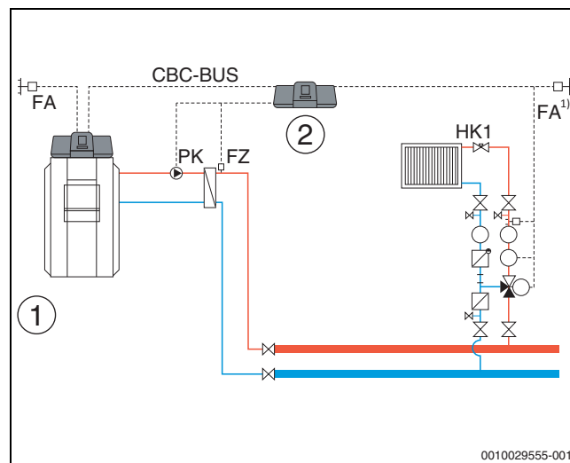
Рис. 34 Вариант 2: система управления низшего уровня с компенсацией потери тепла по датчику FZ и ограничением нагрузки
