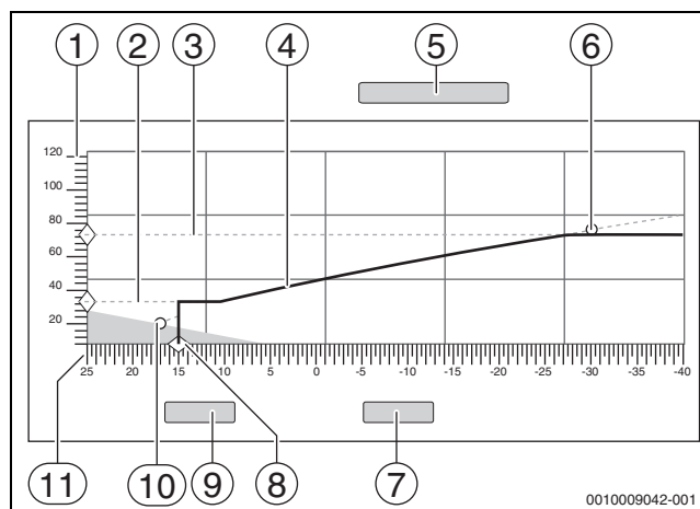
Рис. 43 Отопительная кривая
