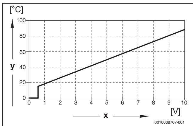
Рис. 28 Вход 0 ... 10 В Температура
