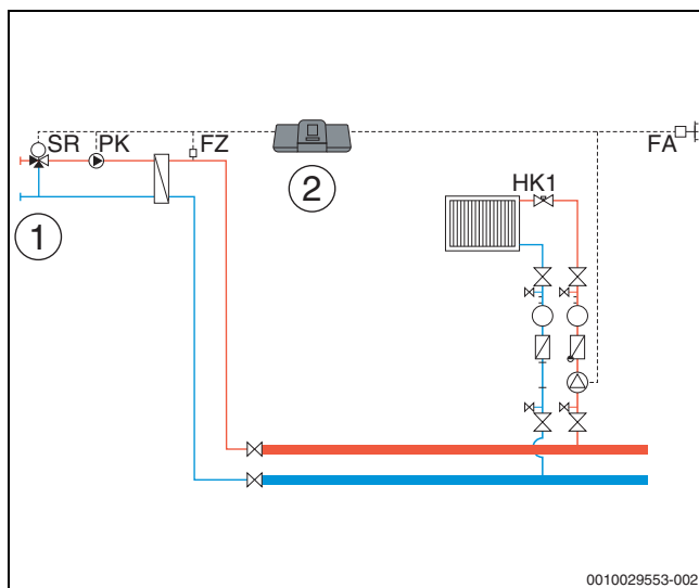
Рис. 32 Вариант 3: сторонний источник тепла без питающего насоса, ограничения нагрузки, функции предварительного смешивания и компенсации потери тепла посредством FZ
