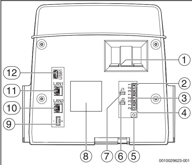
Рис. 23 Задняя сторона пульта управления
