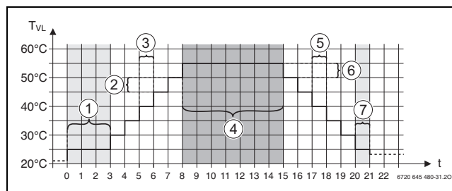
Рис. 44 Сушка монолитного пола
