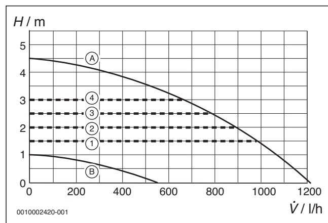
Сурет 87 Жылыту сорғысының әмбебап сипаттамалары мен кестелері
