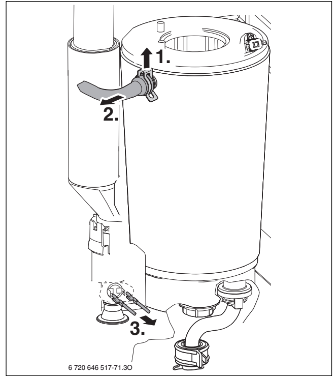
Сурет 80 Жіберу түтігін бұрап, кабельді ажыратыңыз
