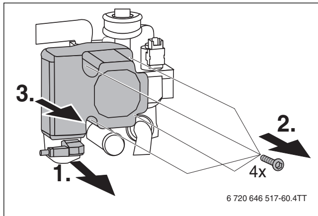
Сурет 75 Жылыту жүйесінің циркуляциялық сорғысын демонтаждаңыз
