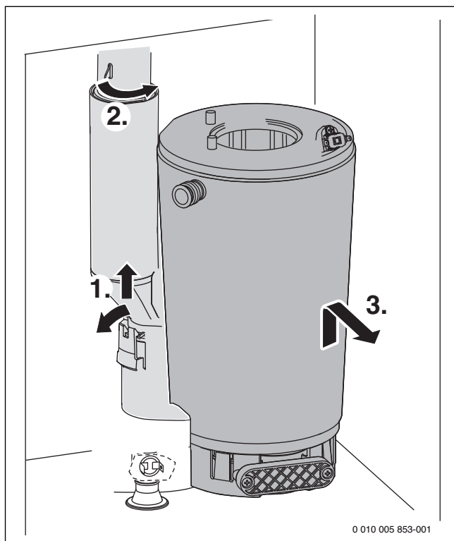
Сурет 82 Жылыту блогын демонтаждаңыз
