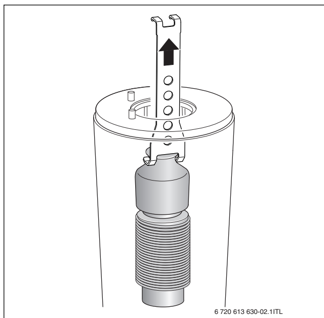
Сурет 59 Жоғарғы сүйір корпусты шығарып алыңыз
