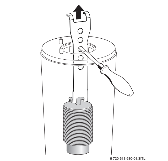
Сурет 60 Төменгі сүйір корпусты шығарып алыңыз
