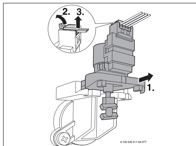
Сурет 70 3-жүрісті қақпақшаның қозғалтқышын шешу
