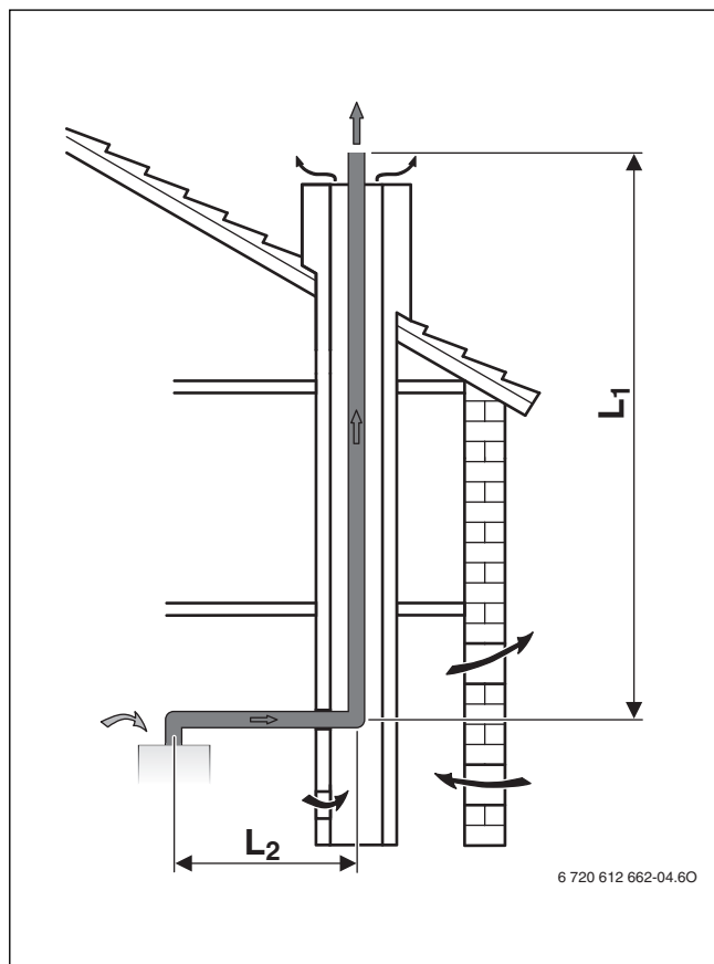
Сурет 7 В 23р бойынша шахтадағы мұржа
