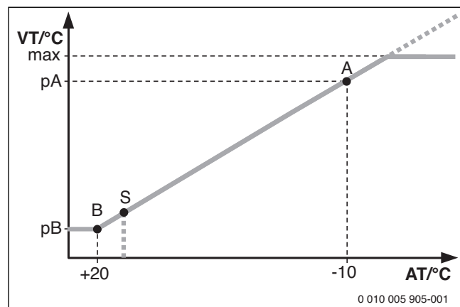
Сурет 86 Қыздыру ауытқымасы
