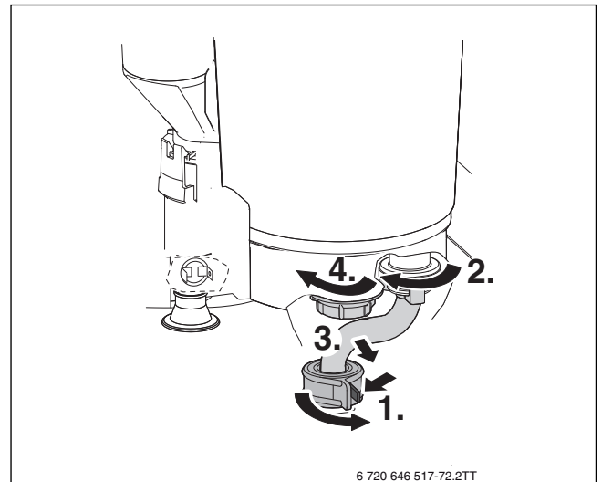
Сурет 81 Гайканы алып, бұрғыш түтікті бұрыңыз
