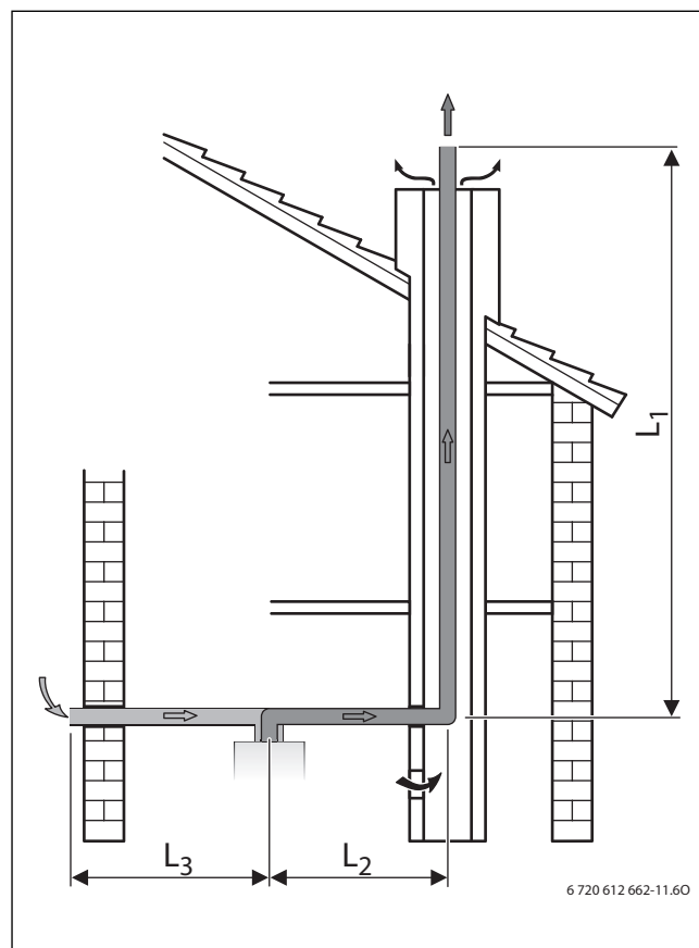
Сурет 11 С 53 бойынша шахтадағы пайдаланылған газ мұржа
