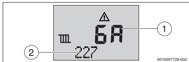
Сурет 81 Мысал: Блоктаушы ақаудың индикациясы
