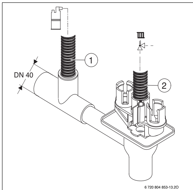
Сурет 28 Конденсатты бұруға арналған шлангіні сифондағы сақтандырғыш клапан шлангісін орнату
