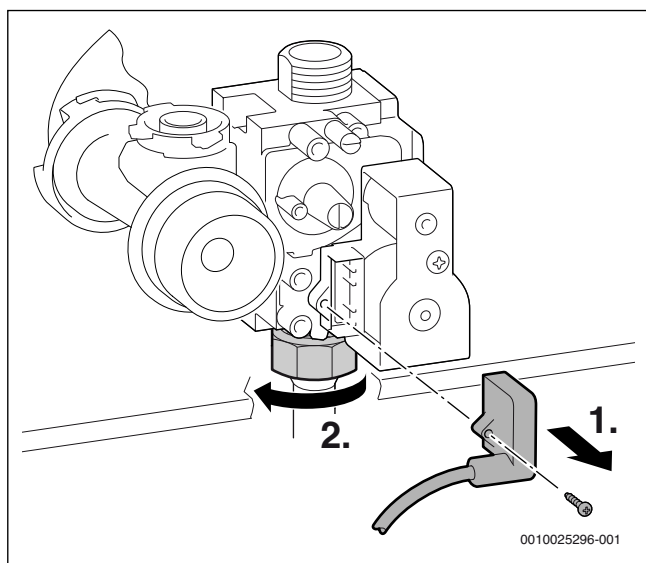
Сурет 74 Штекерді алып шығып, салмалы сомынды босатыңыз
