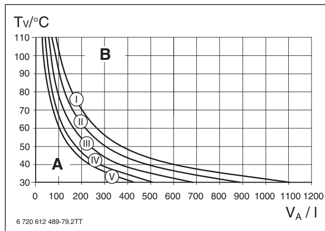
Сурет 23 Кеңейткіш ыдыстың графикалық сипаттары
