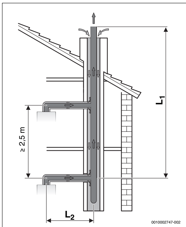
Сурет 19 C_{43x} бойынша концентрациялық тұрбдан көп рет пайдалану
