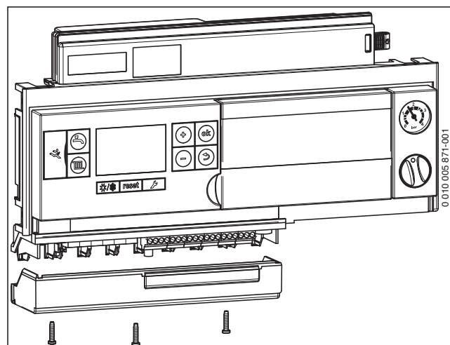
Сурет 32 Қаптамаларды алу
