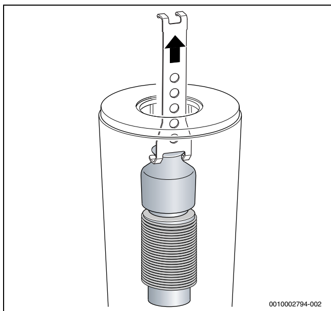
Сурет 59 Жоғарғы сүйір корпусты шығарып алыңыз
