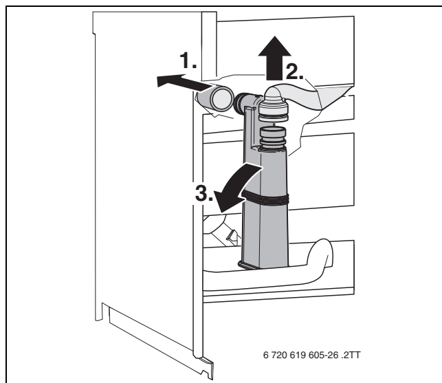
Сурет 64 Конденсат сифонын шешіп алу
