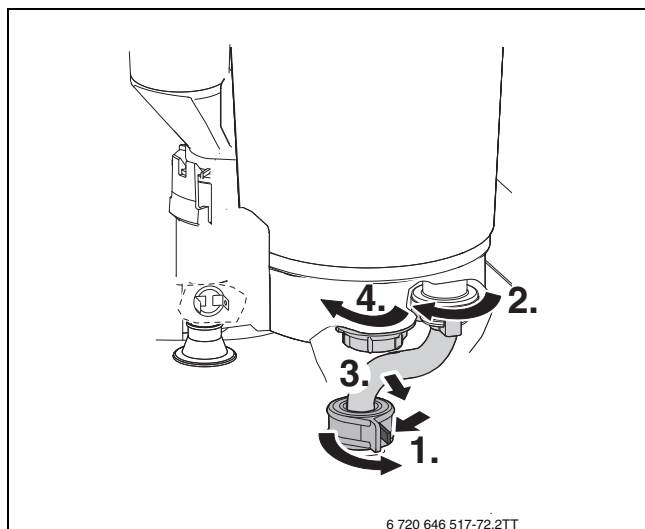
Сурет 80 Гайканы алып, бұрғыш түтікті бұрыңыз
