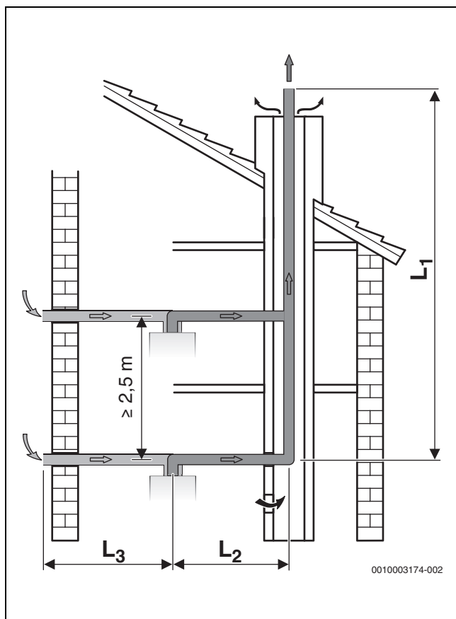
Сурет 19 C_{83} бойынша жеке құбырдан бірнеше көп рет пайдалану
