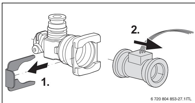
Сурет 68 Суық су құбыр желісіндегі турбинаны демонтаждау
