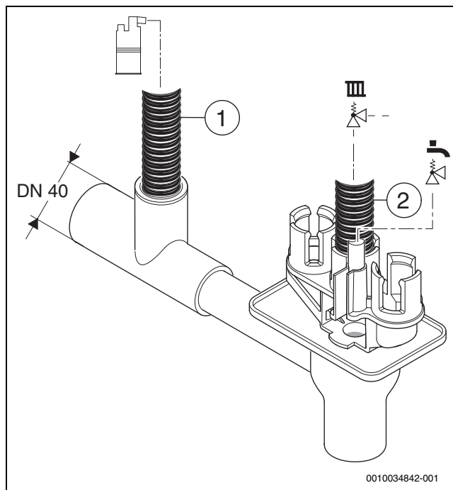
Сурет 27 Конденсат шлангісі мен сақтық клапанының шлангісін сифонға орнатыңыз
