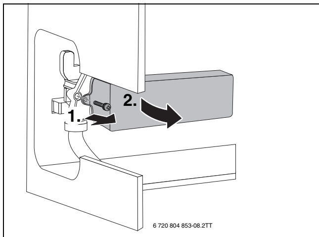
Сурет 66 Пластиналы жылу алмастырғышты демонтаждау
