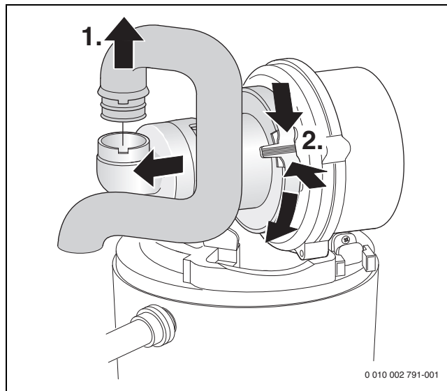
Сурет 56 Сорғыш түтік пен араластырғышты демонтаждаңыз
