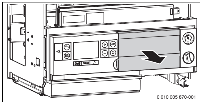
Сурет 30 Қаптаманы алу және басқару блогын құрастыру
