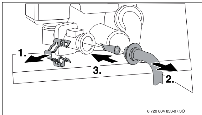
Сурет 67 Суық су құбырындағы електі демонтаждау
