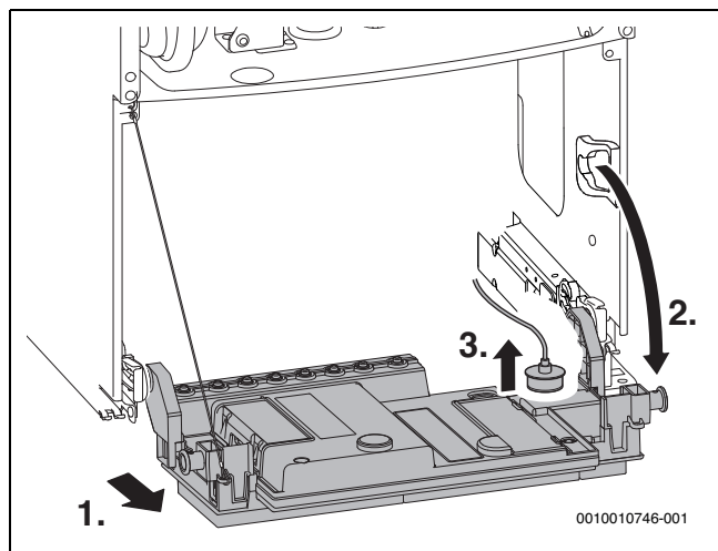
Сурет 76 Басқару блогын төмен түсіріңіз
