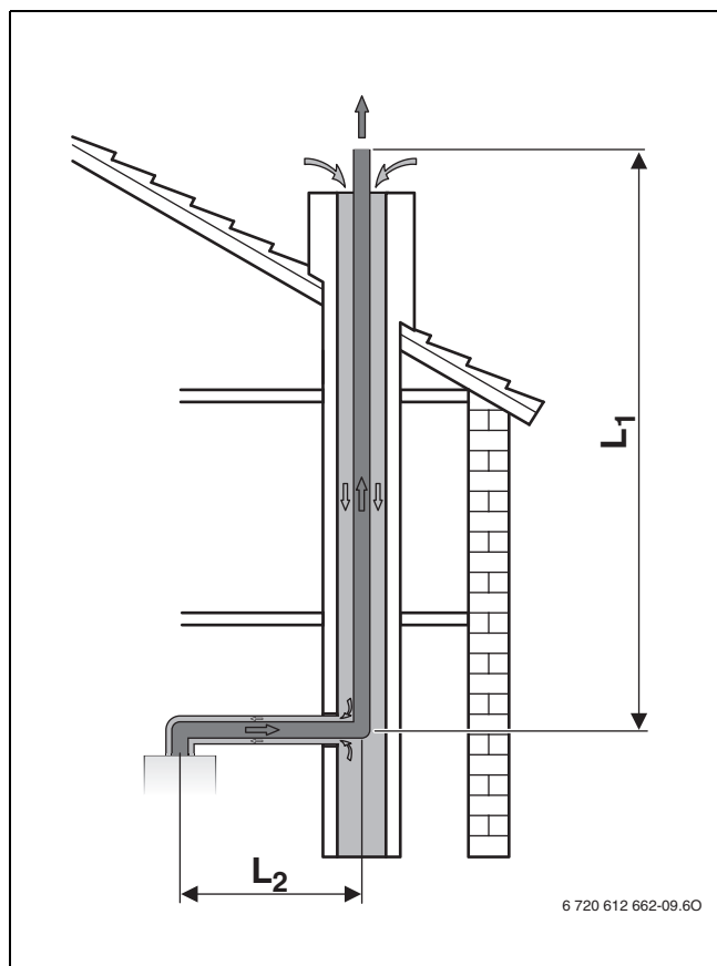
Сурет 11 C 93 бойынша шахтадағы пайдаланылған газ мұржа
