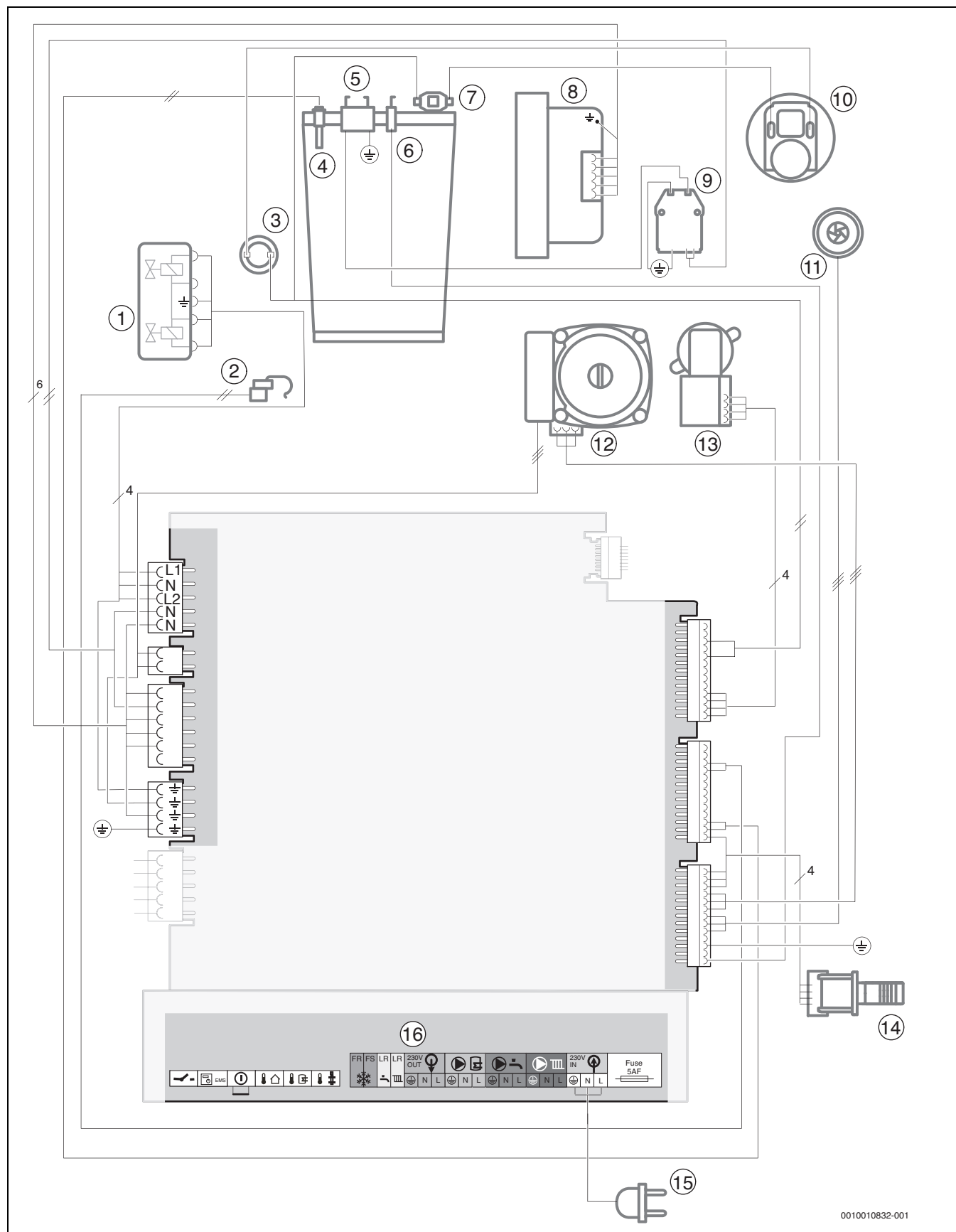
Сурет 84 Электр сымдары
