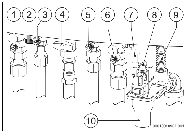
Сурет 28 Газ бен су беру жағына арналған жалғаулар (керек-жарақ)
