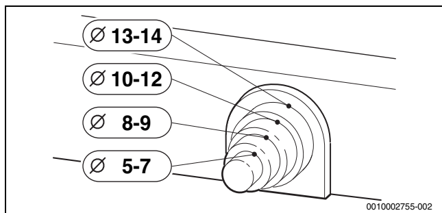
Сурет 32 Кабель кірісін кабель диаметріне келтіру
