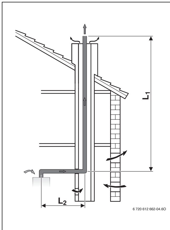
Сурет 7 B 23P бойынша шахтадағы мұржа
