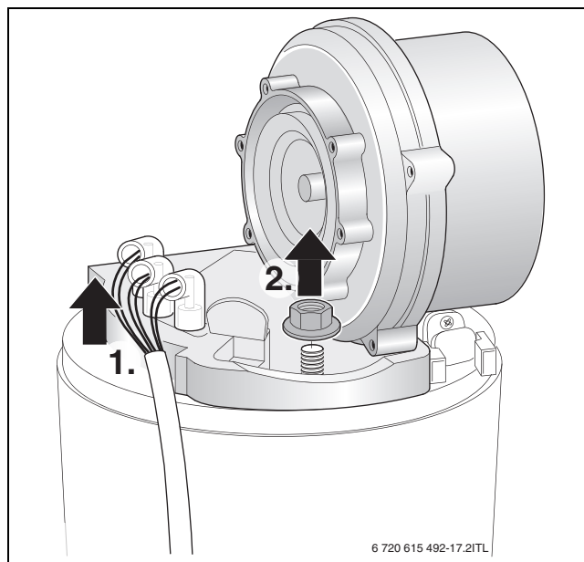
Сурет 57 Ауа үрлегішті шығарып алыңыз
