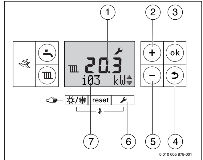
Сурет 46 Басқару элементтеріне шолу
