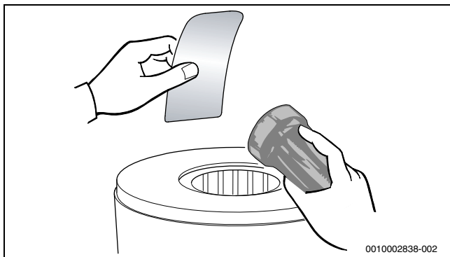
Сурет 62 Жылыту блогында қалдық қалмағанын тексеріңіз
