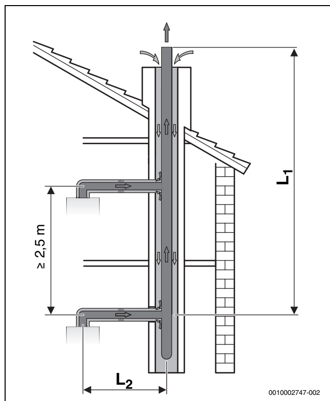
Сурет 18 C 43 бойынша концентрациялық құбырдан бірнеше көп рет пайдалану
