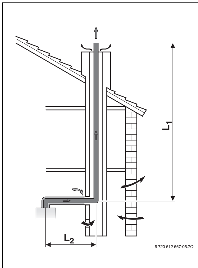
Сурет 8 B 33 бойынша шахтадағы мұржа
