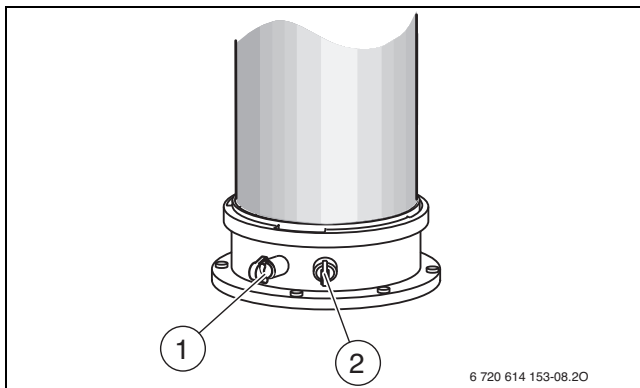
Сурет 54 Пайдаланылған газдар мен жанатын ауаны өлшеуге арналған штуцер
