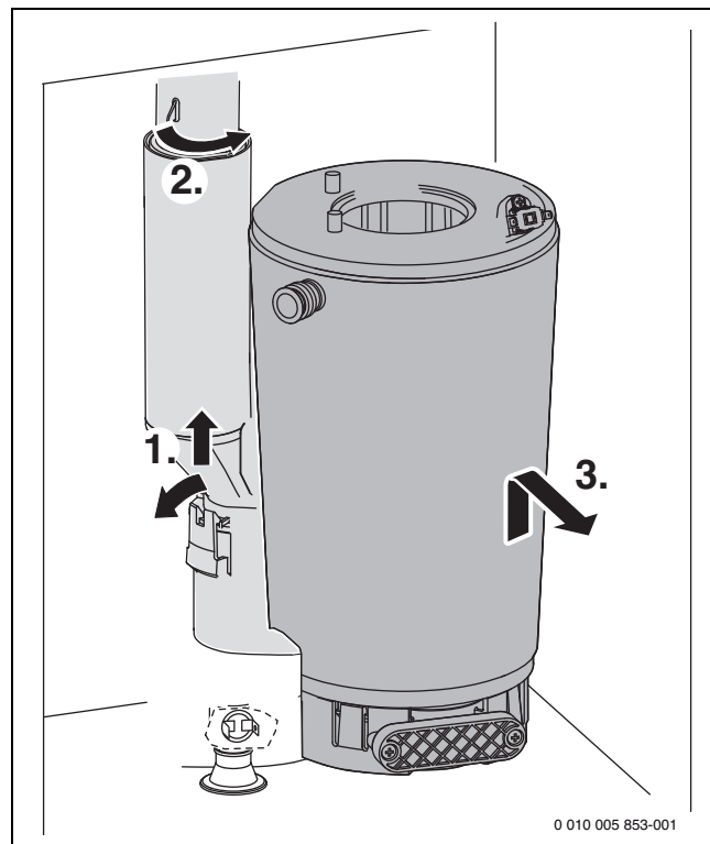
Сурет 81 Жылыту блогын демонтаждаңыз
