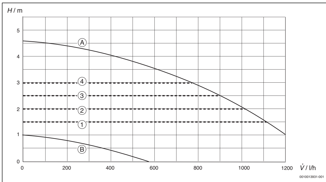
Сурет 86 Жылыту сорғысының әмбебап сипаттамалары мен кестелері
