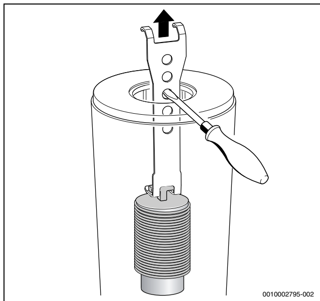
Сурет 60 Төменгі сүйір корпусты шығарып алыңыз
