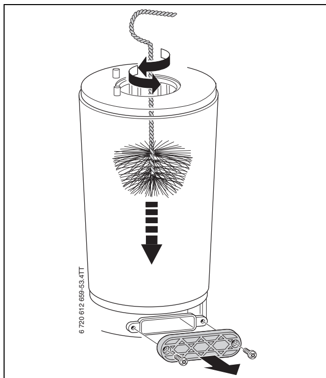
Сурет 61 Жылыту блогын тазалаңыз
