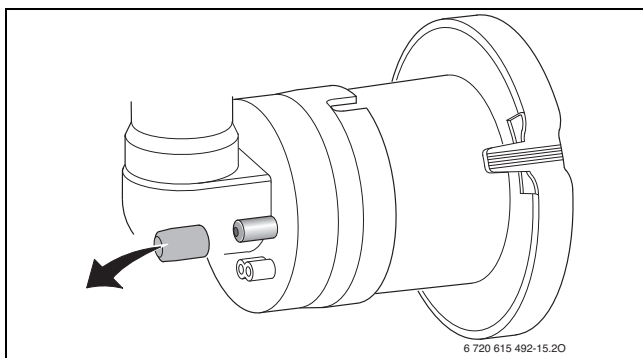
Сурет 55 Араластырғыштағы өлшегіш штуцер
